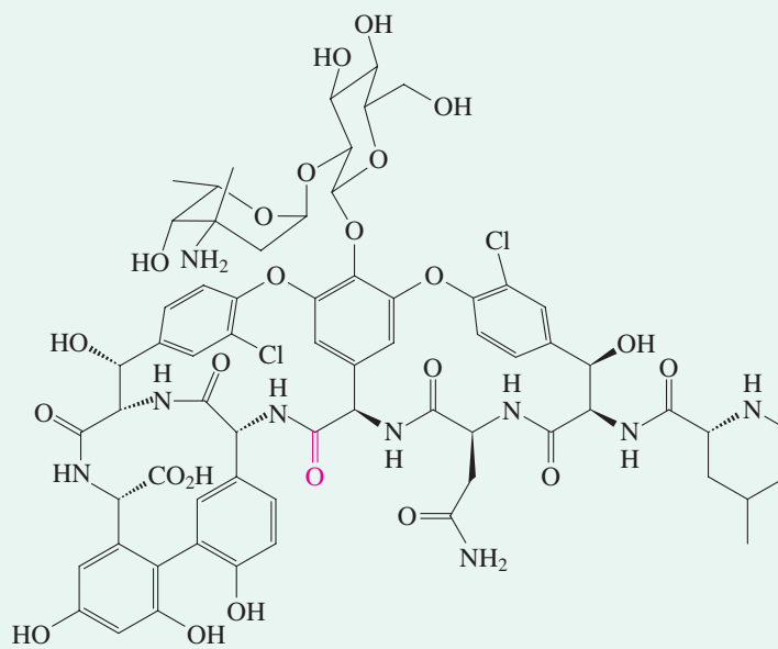
Vancomycin
