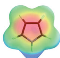
Pyrrole
