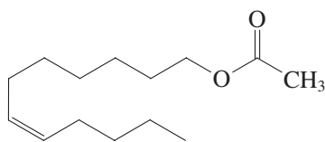
(Z)-7-Dodecenyl acetate
