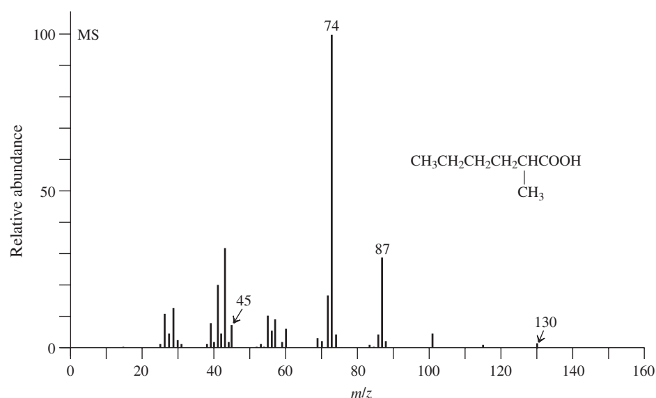
MS-H
