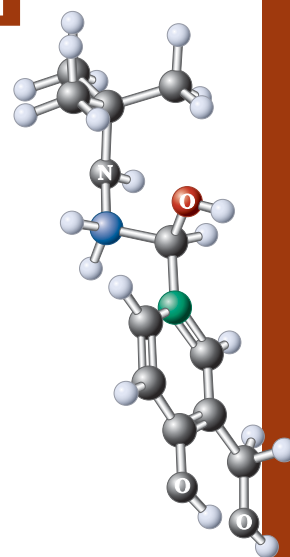
S-(+)-Albuterol
