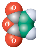
2-Butenedioic anhydride (Maleic anhydride)
