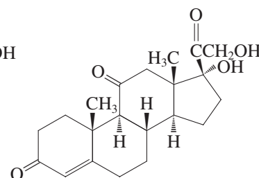
Cortisone
