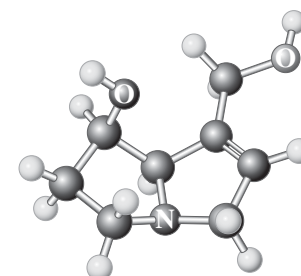
Retronecine
