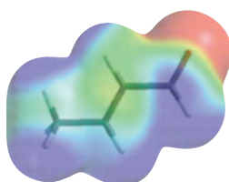
2-Butenal
