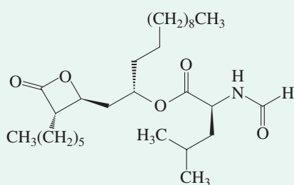
Orlistat (Xenical)
