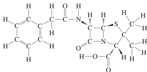
Benzylpenicillin
