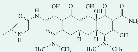
Tigecycline (Tygacil)
