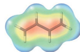
1,3-Butadiene (Conjugated)
