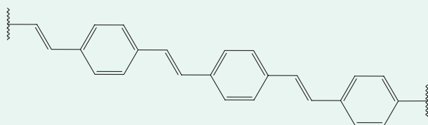
Poly( p -phenylene vinylene)
