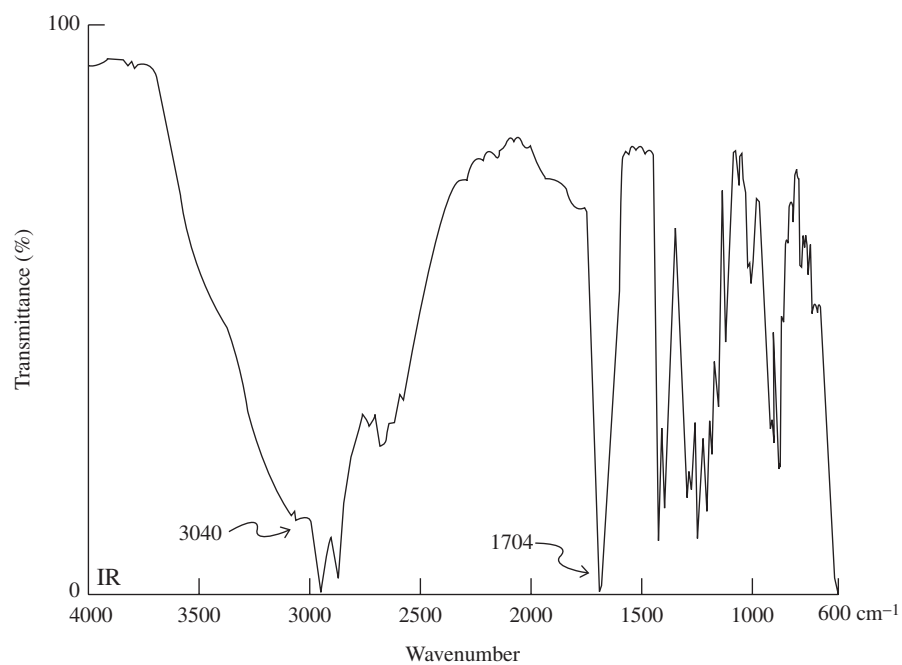
IR-A
