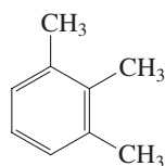
1,2,3-Trimethylbenzene
