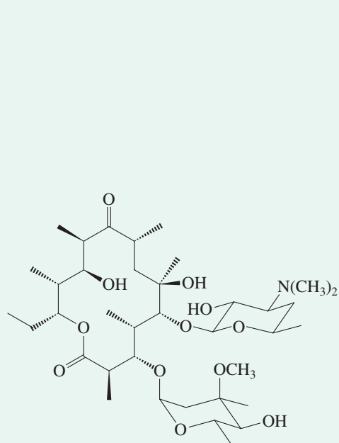
Erythromycin
